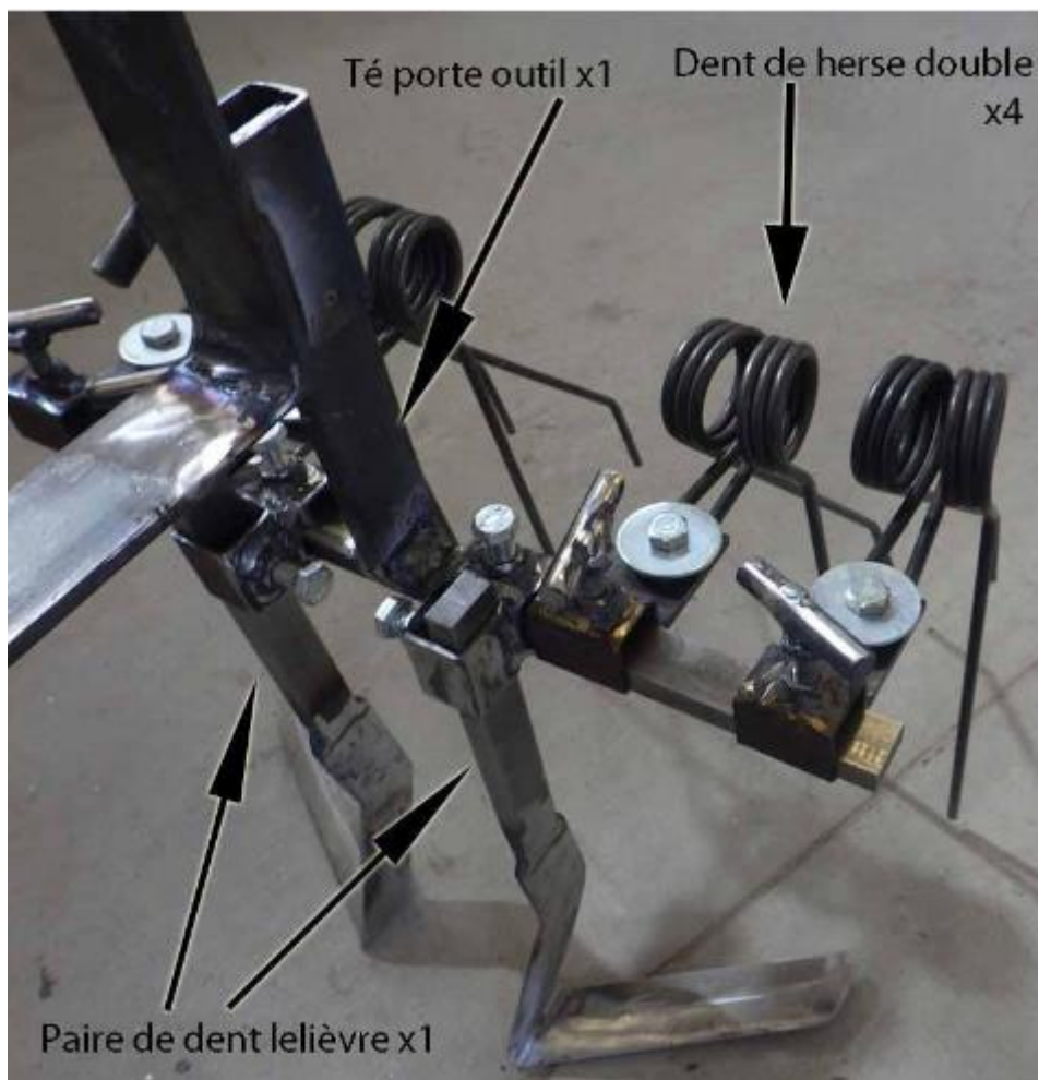
Figure 10 : Exemple de combinaison d'outils sur la houe maraîchère
