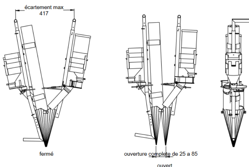
Figure 19 : Aperçu de la canne à planter de l'Atelier Paysan
