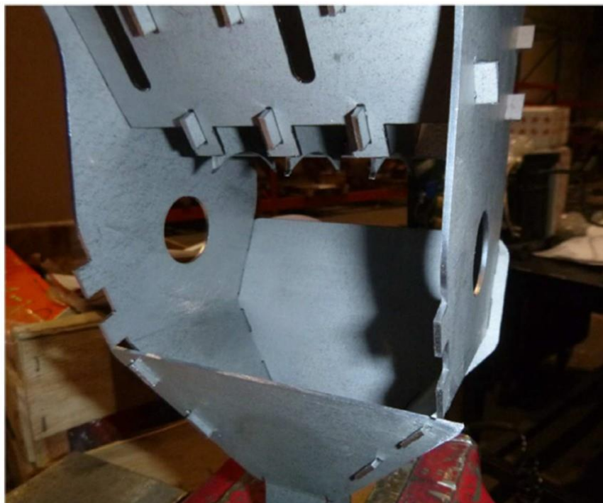
Figure 39 : Le distributeur de graines : assemblage par tenon mortaise sans soudure
