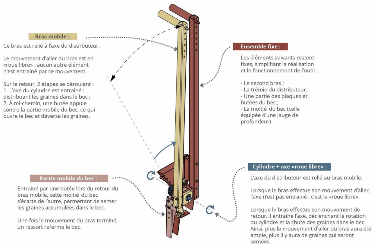
Figure 27 : Mobilité des parties de la canne à semer
