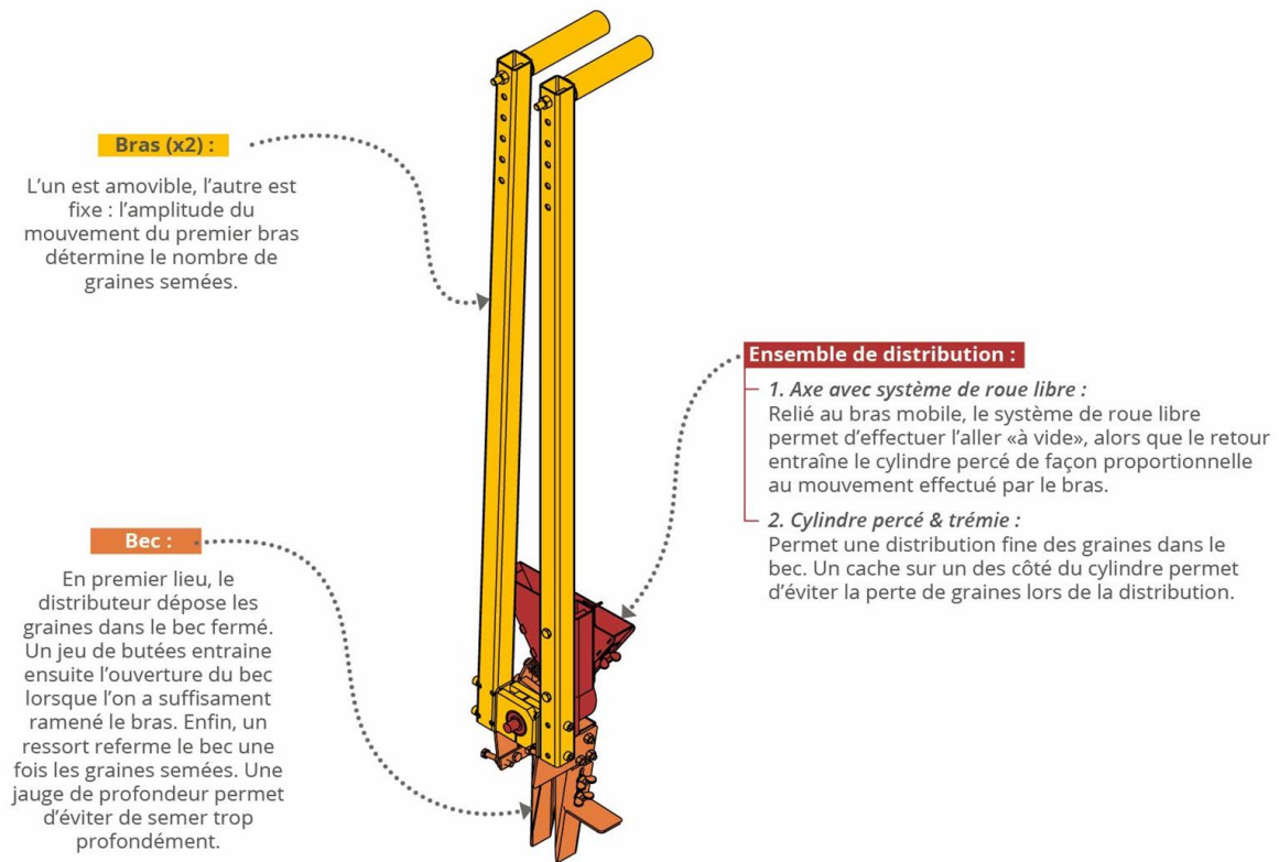
Figure 26 : Fonctions des éléments de la canne à semer de l'Atelier Paysan
