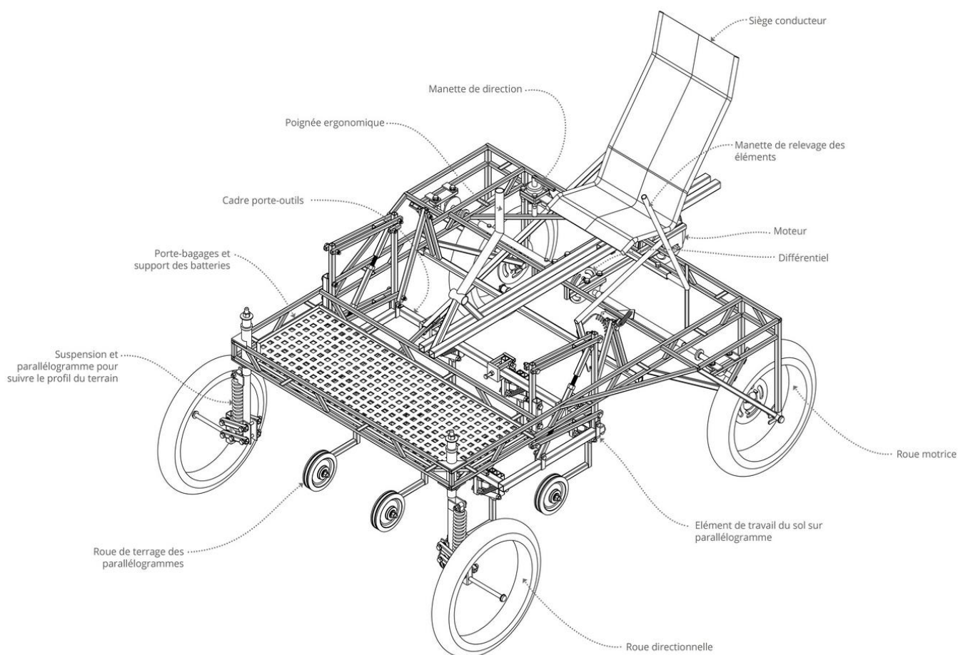
Figure 84 : Schéma de l'Aggrozouk
